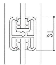
中棧形状 (中棧のある場合)
